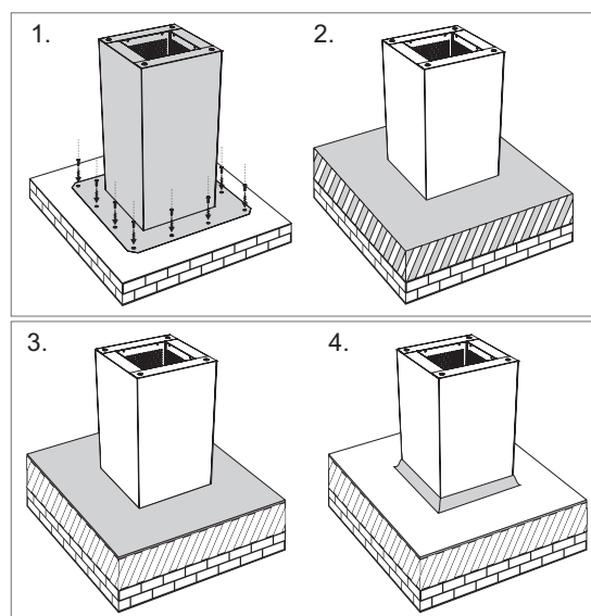
Afbeelding 5.5.20 Schoorsteen installatie
