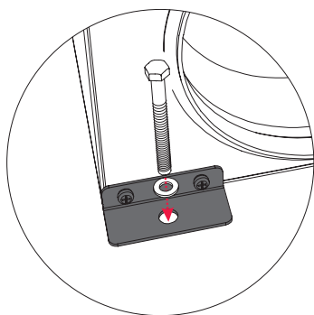
Afbeelding 5.5.5 Montage
