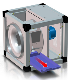
Afbeelding 5.5.10 Houd bij het aansluiten van luchtkanalen rekening met de luchtstroomrichting aangegeven op de behuizing van het toestel.
