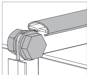
Afbeelding 5.5.13 Ventilatoraansluiting middels bouten en een C-profiel
