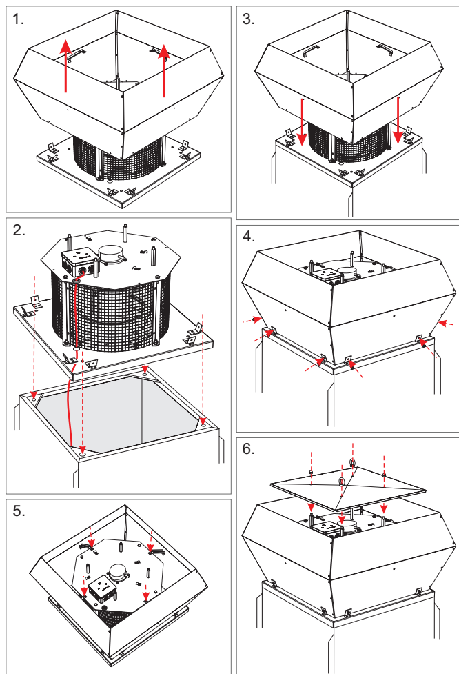
Afbeelding 5.5.25 Montage
