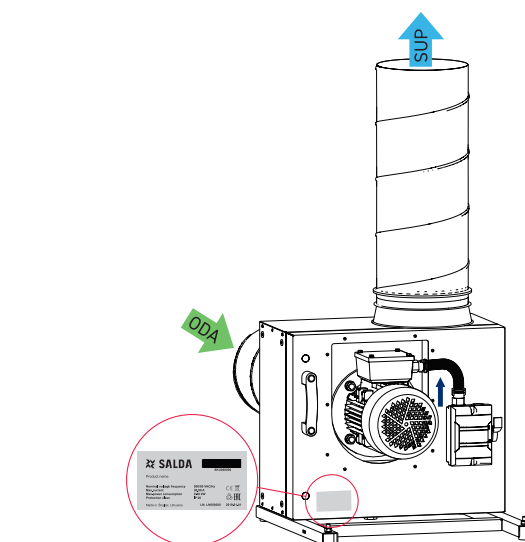
Afbeelding 2.5 KF T120 / KF T120 plek van het technisch label en richting van de luchtstroom
