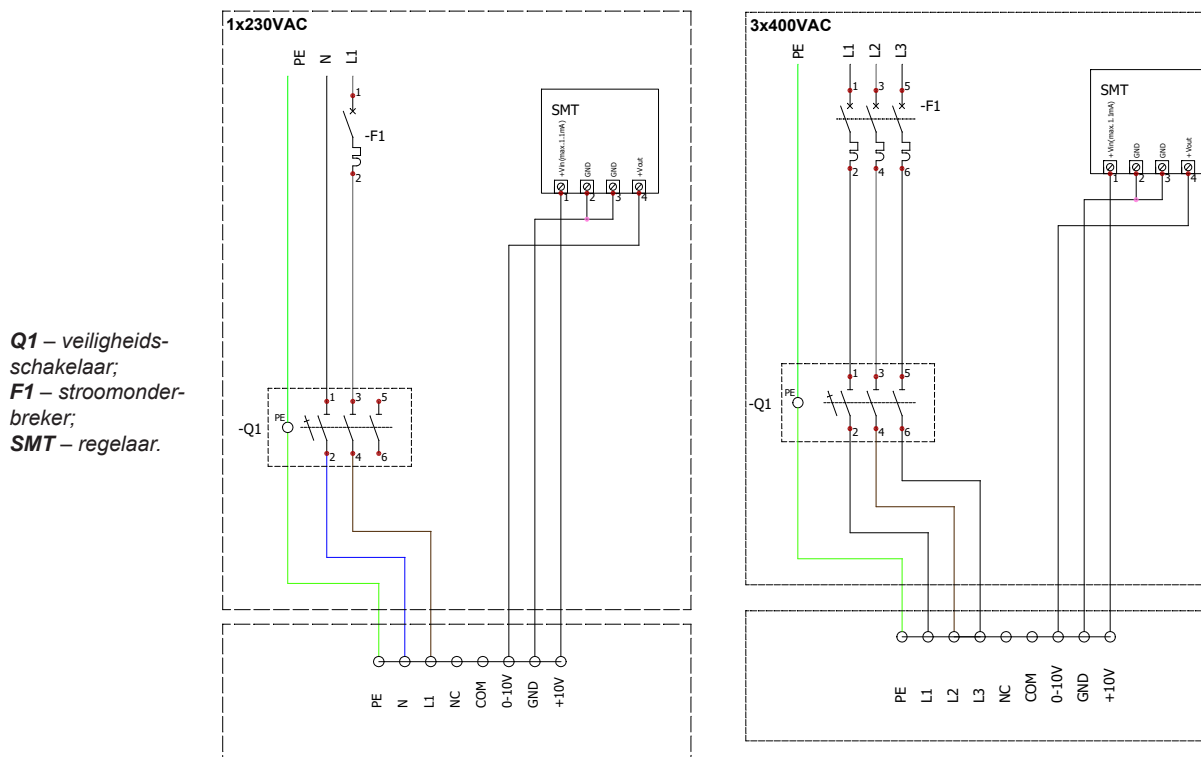
Afbeelding 8.1.2 SMT-pinout en aansluitvoorbeeld
