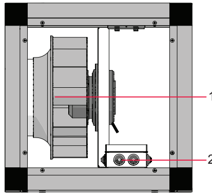
Afbeelding 4.6.5 KUB EKO
