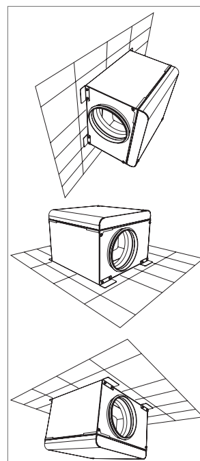
Afbeelding 5.5.2 Installatie aan de muur, vloer of plafond
