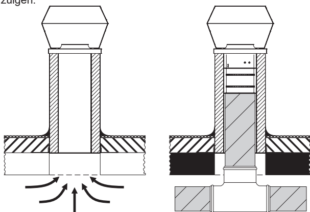
Afbeelding 5.5.19 Aansluiting van het luchtkanaal
