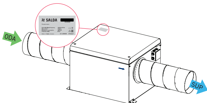
Afbeelding 2.4 AKU / AKU EKO plek van het technisch label en richting van de luchtstroom
