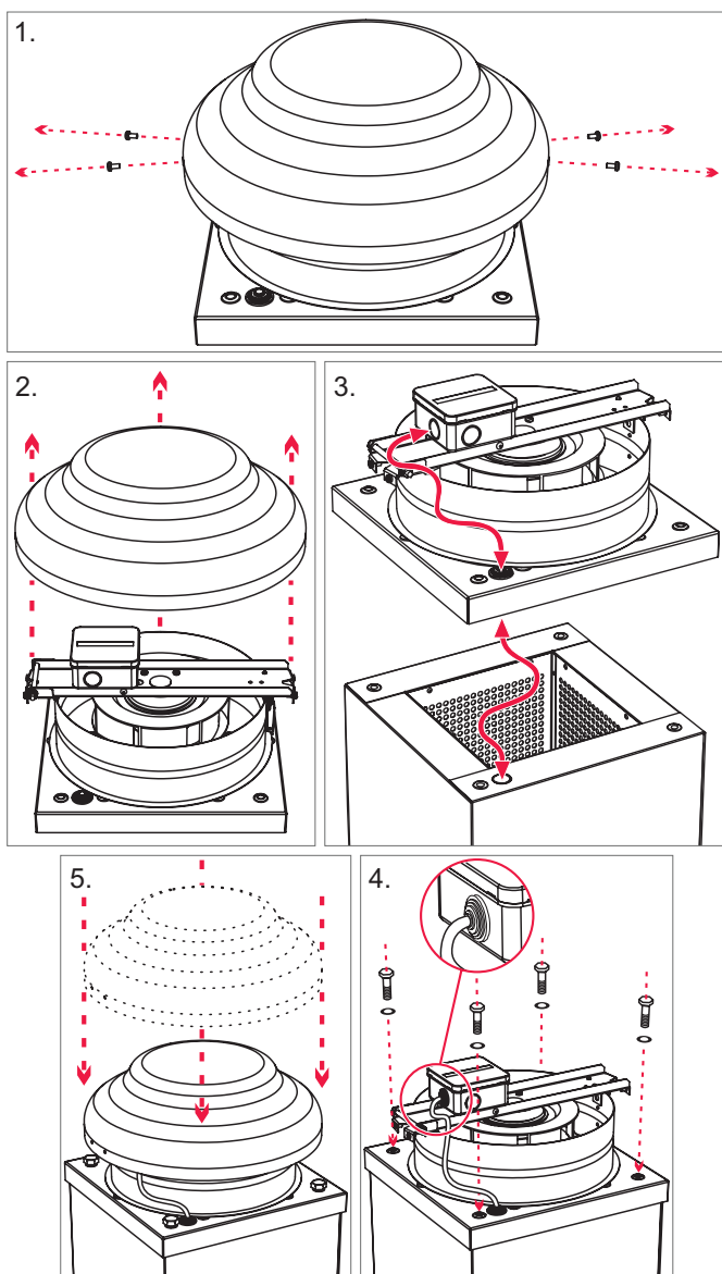
Afbeelding 5.5.21 Montage en installatie met behulp van accessoires
