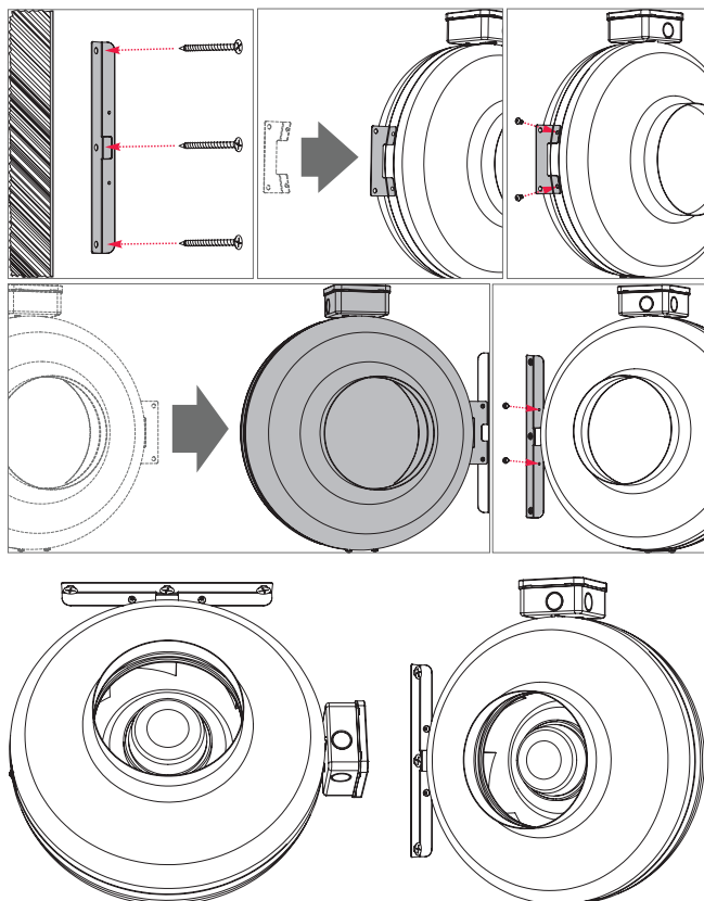
Afbeelding 5.5.11 Bevestiging van het apparaat aan de muur met behulp van het steunelement
