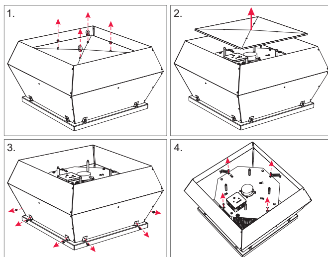
Afbeelding 5.5.24 Openen panelen
