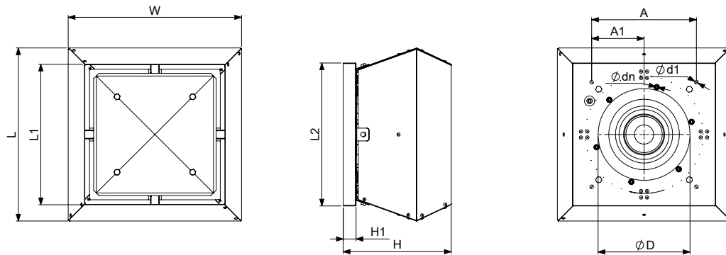
Afbeelding 4.2.9 VSV / VSV AL / VSV AL EKO
