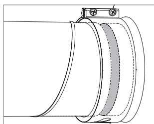
Afbeelding 5.5.17 Montage met speciale accessoires – adapters
