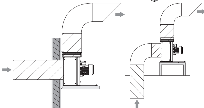
Afbeelding 5.5.6 Vervanging van de onderhoudsdeurzijde van de ventilator
