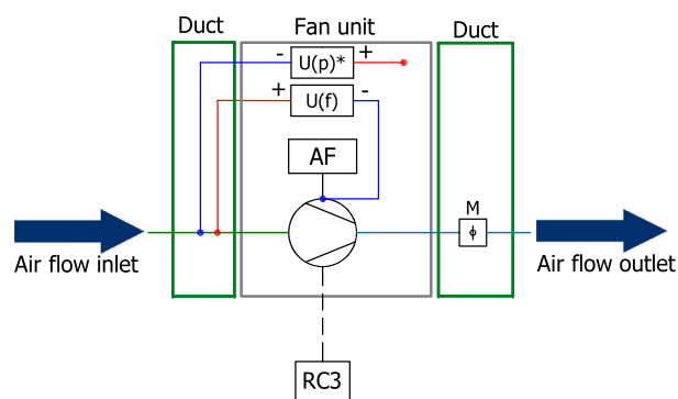
Afbeelding 5.4.2 VSVI EKO AL CPG Ventilatoren
