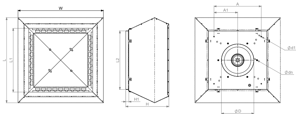
Afbeelding 4.2.10 VSVI / VSVI AL / VSVI AL EKO
