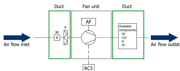
Afbeelding 5.4.4 AKU, AKU EKO, VKAP 3.0, VKA EKO, VKS, VKSA Ventilatoren
