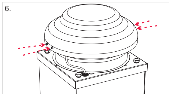
Afbeelding 5.5.22 Montage
