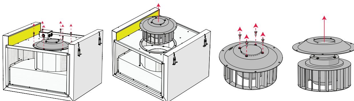
Afbeelding 6.4.4 VKS / VKSA
