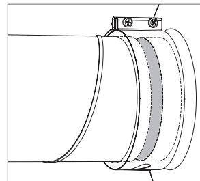
Afbeelding 5.5.1 Klembevestiging
