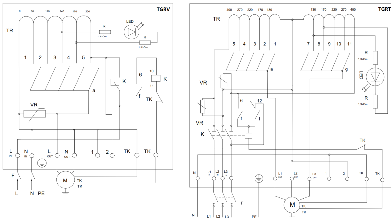
Afbeelding 8.2.2 TRGV / TRGT pinout en aansluitvoorbeeld
