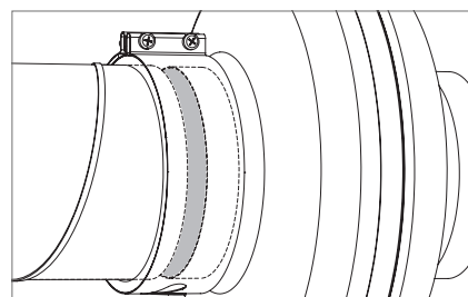
Afbeelding 5.5.12 Aansluiting op het kanaal met behulp van de klem
