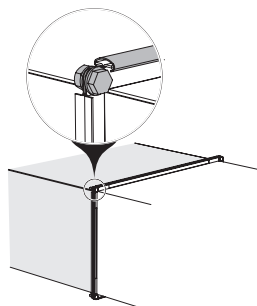
Afbeelding 5.5.9 Trilling-sisolerende pakking
