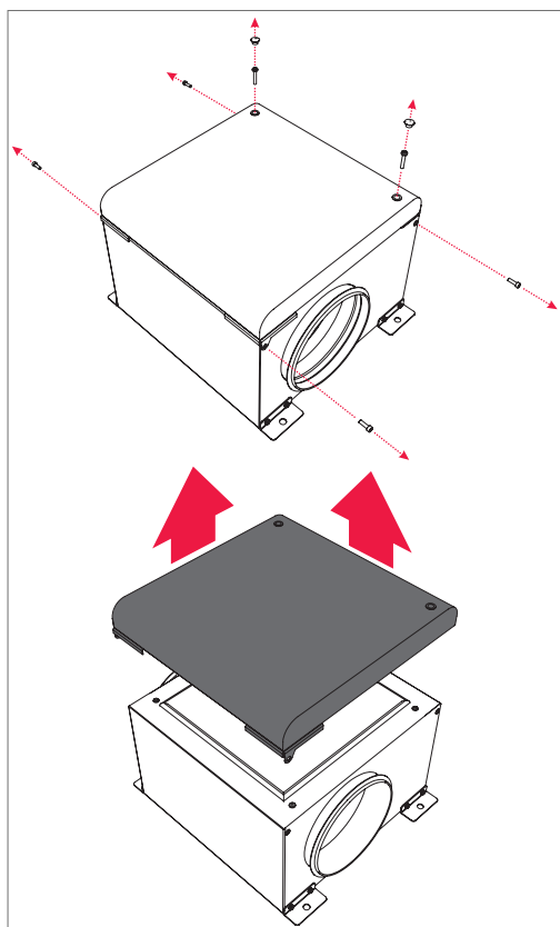
Afbeelding 5.5.6 Vervanging van de onderhoudsdeurzijde van de ventilator
