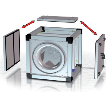
Afbeelding 5.5.8 De onderhoudskant veranderen
