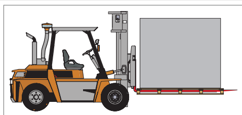
Afbeelding 5.2.1 Hijsen d.m.v. vorkhefift
