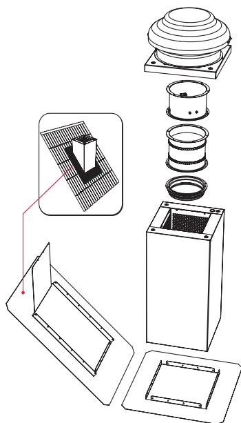
Afbeelding 5.5.21 Montage en installatie met behulp van accessoires
