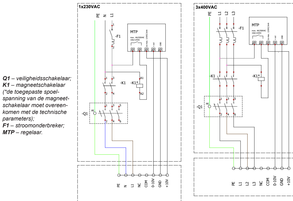
Afbeelding 8.1.1 MTP-pinout en verbindingvoorbeeld
