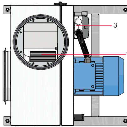
Afbeelding 4.6.2 KF T120
