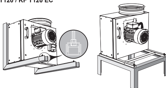
Afbeelding 5.5.7 Vervanging van de onderhoudsdeurzijde van de ventilator
