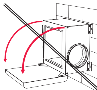
Afbeelding 5.5.3 Onjuiste ventilatorinstallatie
