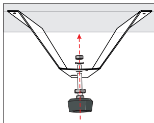
Figuur 5.5.2.1 Vloermontage
