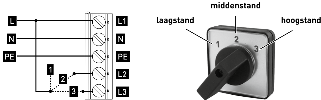
Figuur 10: Perilex-schakelaar
