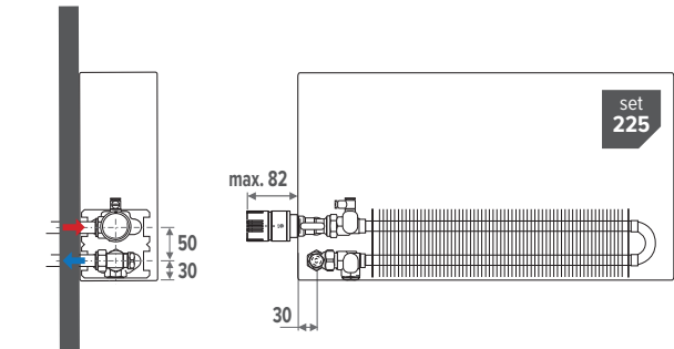
Voorbeeld aansluiting links
