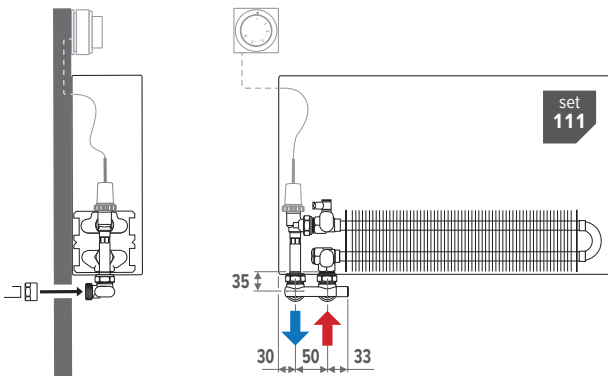
Voorbeeld aansluiting links
