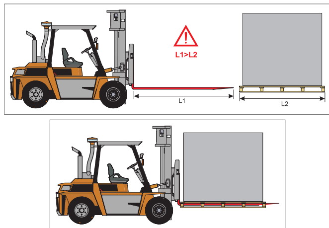
Afbeelding 5.2.1 Hijsen d.m.v. vorkhefift
