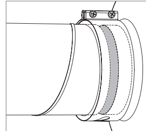
Afbeelding 5.5.1 Klembevestiging
