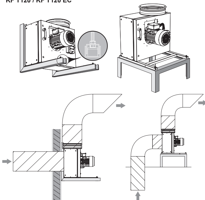
Afbeelding 5.5.6 Vervanging van de onderhoudsdeurzijde van de ventilator
