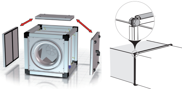
Afbeelding 5.5.8 De onderhoudskant veranderen
