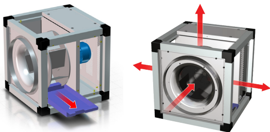
Afbeelding 5.5.10 Houd bij het aansluiten van luchtkanalen rekening met de luchtstroomrichting aangegeven op de behuizing van het toestel.
