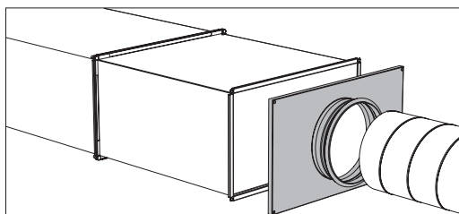
Afbeelding 5.5.18 Er moet voldoende ruimte worden vrijgehouden voor het openen en reinigen van de waaiër
