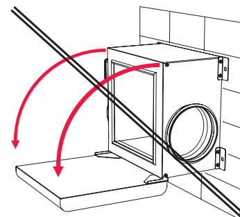
Afbeelding 5.5.3 Onjuiste ventilatorinstallatie
