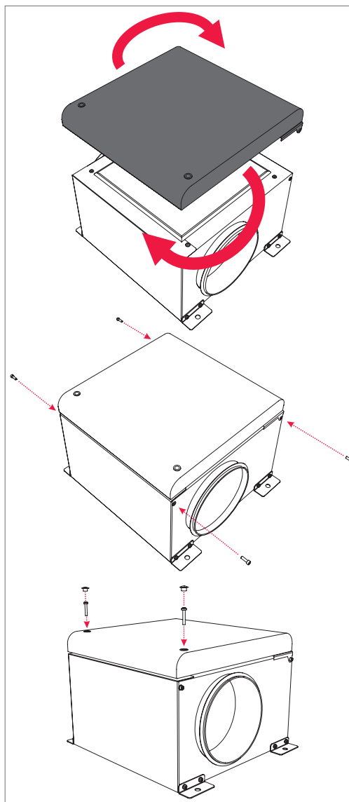
Afbeelding 5.5.7 Vervanging van de onderhoudsdeurzijde van de ventilator
